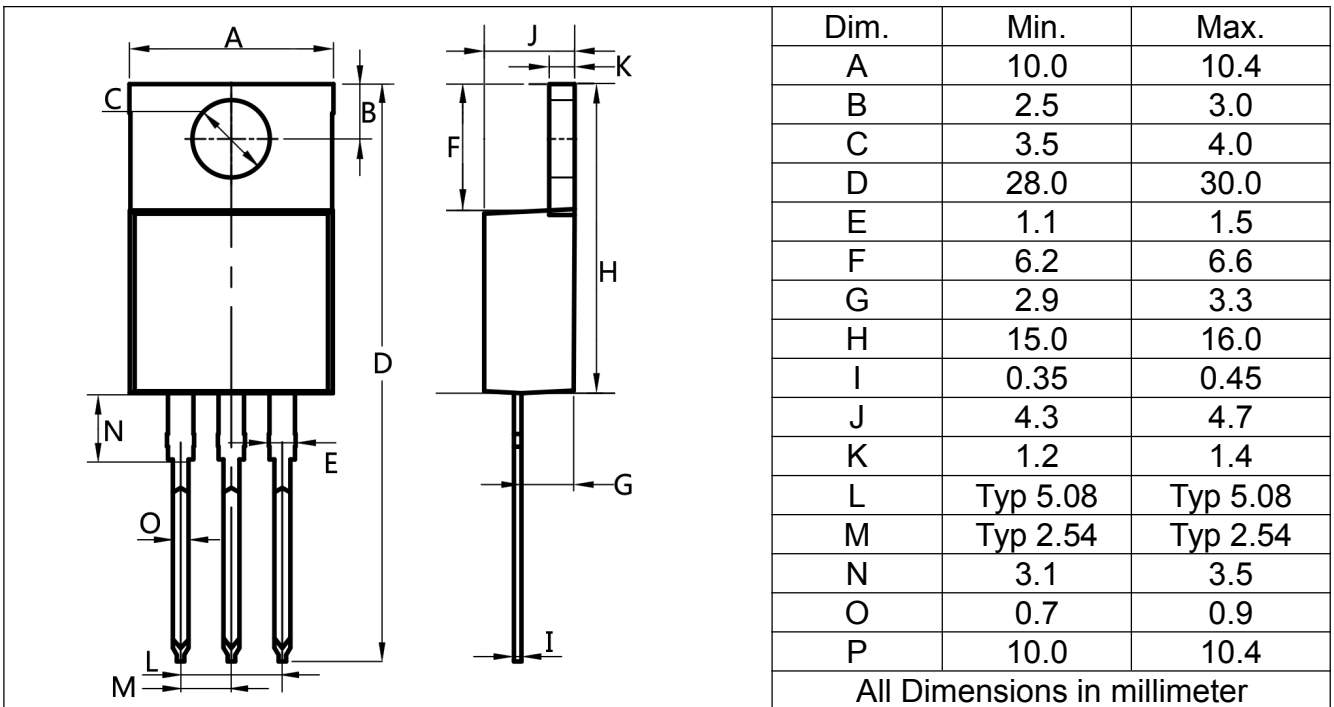
TO-220 封装尺寸 Package size
