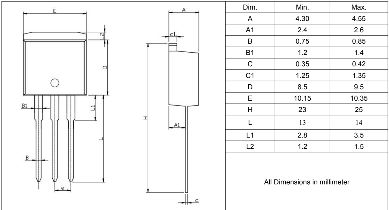
TO-220 封装尺寸 Package size
